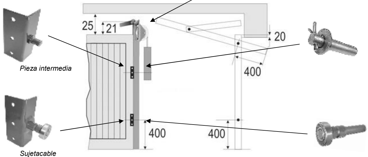
Roldana fija
